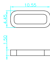
防水圈图示
